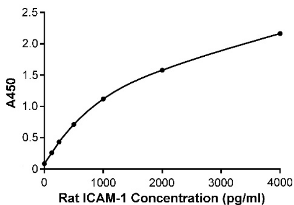
图3. Rat ICAM-1/CD54 ELISA Kit的标准曲线。实测数据会因实验条件、检测仪器等的不同而存在差异，图中数据仅供参考。
